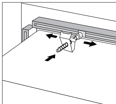
Bottom view of sink Vue du dessous de l'évier Vista inferior del fregadero
